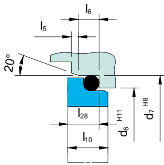
G6 (EN 12756)
